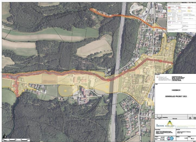
Abbildung 1: Gefahrenzonenkarte im Ortskern von Warth vor der Verbauung
