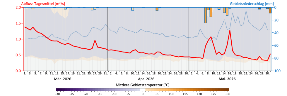
Abbildung 13. Pegel Rohrbach an der Lafnitz und Oberwart. Obere Reihe: Abflussganglinien (Tagesmittel) 2026, langjährige Tagesmittelwerte; innerhalb der blauen Fläche liegen 90 Prozent der Tagesmittel, die orangenen Begrenzungen zeigen die Minima und Maxima. Untere Reihe: vergangene drei Monate mit zusätzlich dargestellten Tagesgebietsniederschlagssummen (Balken) und mittleren täglichen Gebietstemperaturen (Einfärbung Balken) in den Pegelinzugsgebieten.
