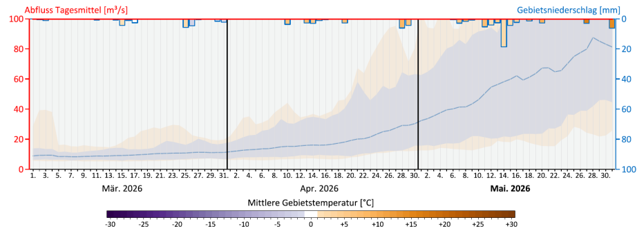
Abbildung 16. Pegel Lienz und Winklarn. Obere Reihe: Abflussganglinien (Tagesmittel) 2026, langjährige Tagesmittelwerte; innerhalb der blauen Fläche liegen 90 Prozent der Tagesmittel, die orangenen Begrenzungen zeigen die Minima und Maxima. Untere Reihe: vergangene drei Monate mit zusätzlich dargestellten Tagesgebietsniederschlags-summen (Balken) und mittleren täglichen Gebietstemperaturen (Einfärbung Balken) in den Pegelinzugsgebieten. Hinweis: Lienz wg. Baumaßnahmen momentan keine Daten!
