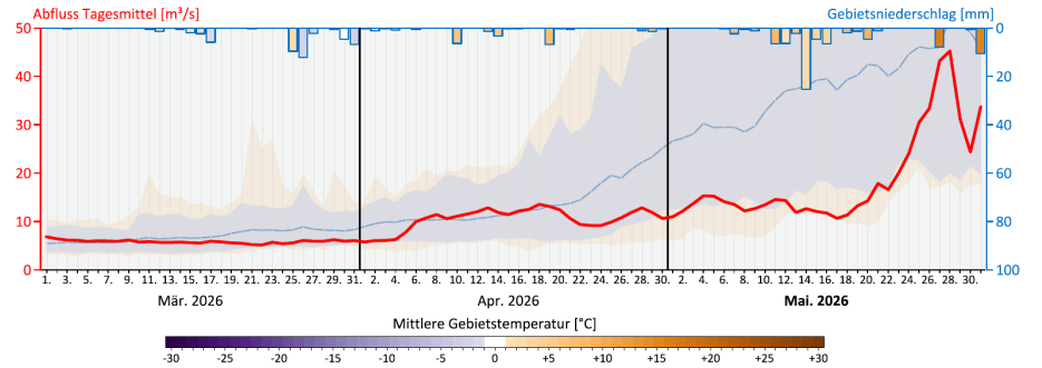
Abbildung 3. Pegel St. Johann in Tirol und Mittersill. Obere Reihe: Abflussganglinien (Tagesmittel) 2026, langjährige Tagesmittelwerte; innerhalb der blauen Fläche liegen 90 Prozent der Tagesmittel, die orangenen Begrenzungen zeigen die Minima und Maxima. Untere Reihe: vergangene drei Monate mit zusätzlich dargestellten Tagesgebietsniederschlagssummen (Balken) und mittleren täglichen Gebietstemperaturen (Einfärbung Balken) in den Pegelinzugsgebieten.
