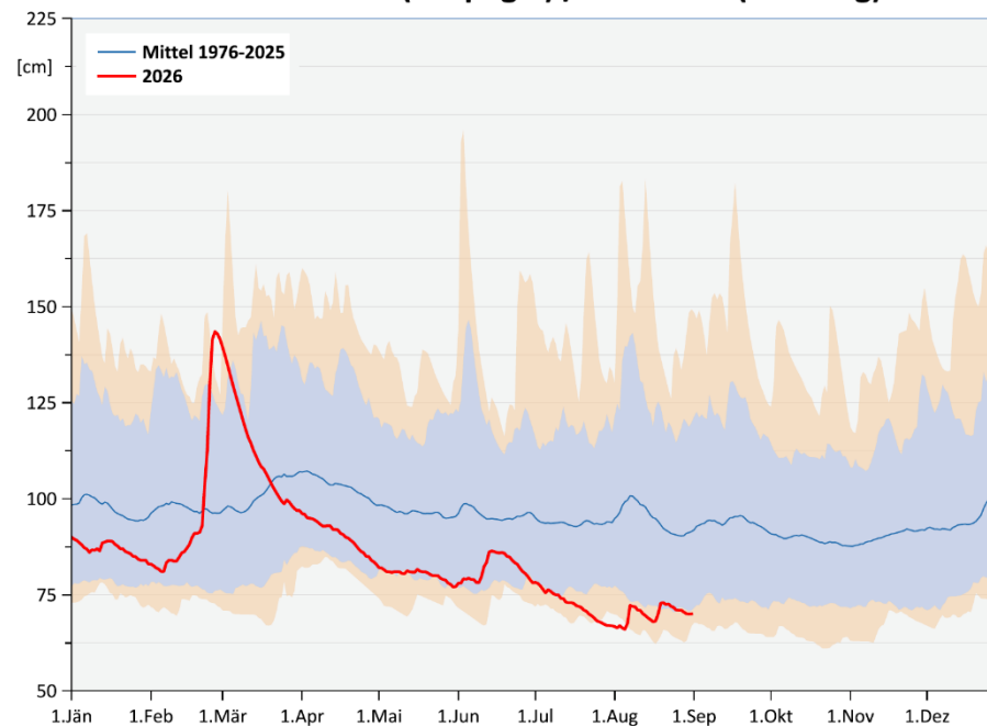
203653 Fuschl (Seepiegel) / Fuschlsee (Salzburg)
