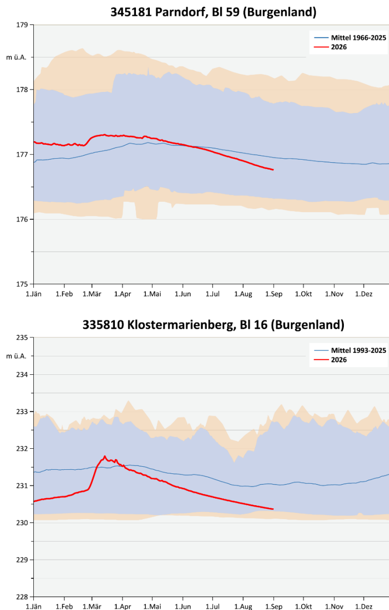
Abbildung 29. Tagesmittel des Grundwasserstandes 2026 (Parndorfer Platte, Seewinkel, Rabnitztal, Raabtal) im Vergleich zum langjährigen Tagesmittel; innerhalb der blauen Fläche liegen 90 Prozent der Tagesmittel, die orangenen Begrenzungen zeigen die Minima und Maxima.
