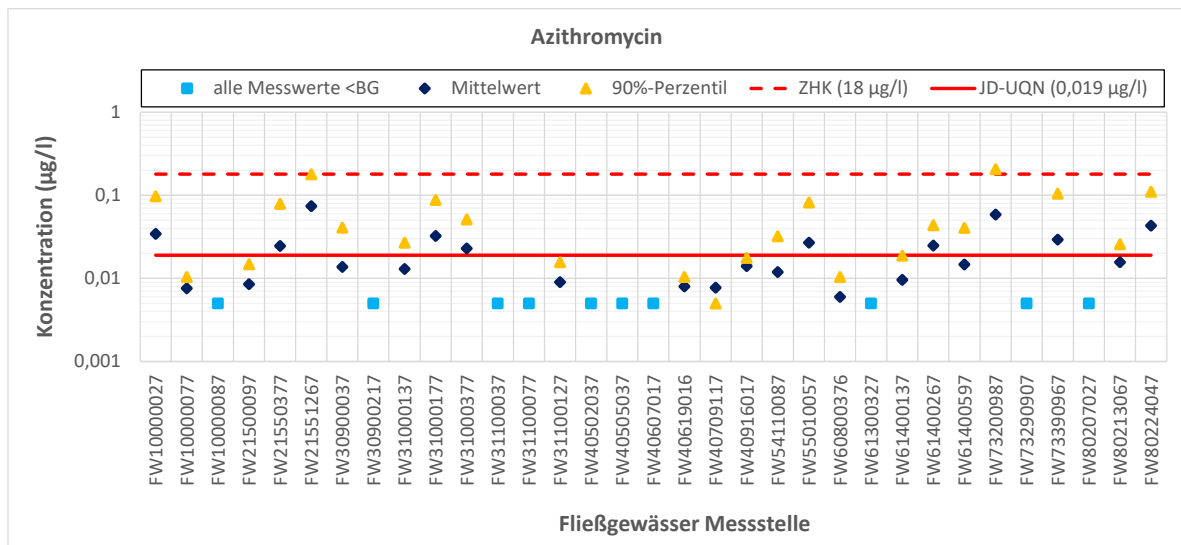
Abbildung 28: Messergebnisse für Azithromycin ( \mu\text{g/l} ) und Gegenüberstellung mit den UQN.
