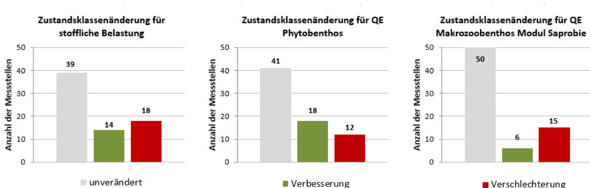
Abbildung 18: Zustandsklassenänderung bei den Überblicksmessstellen an Fließgewässern zwischen den Jahren 2007 (Erstbeobachtung 1. Zyklus) und 2022 (Wiederholungsbeobachtung 3. Zyklus) n=71.
