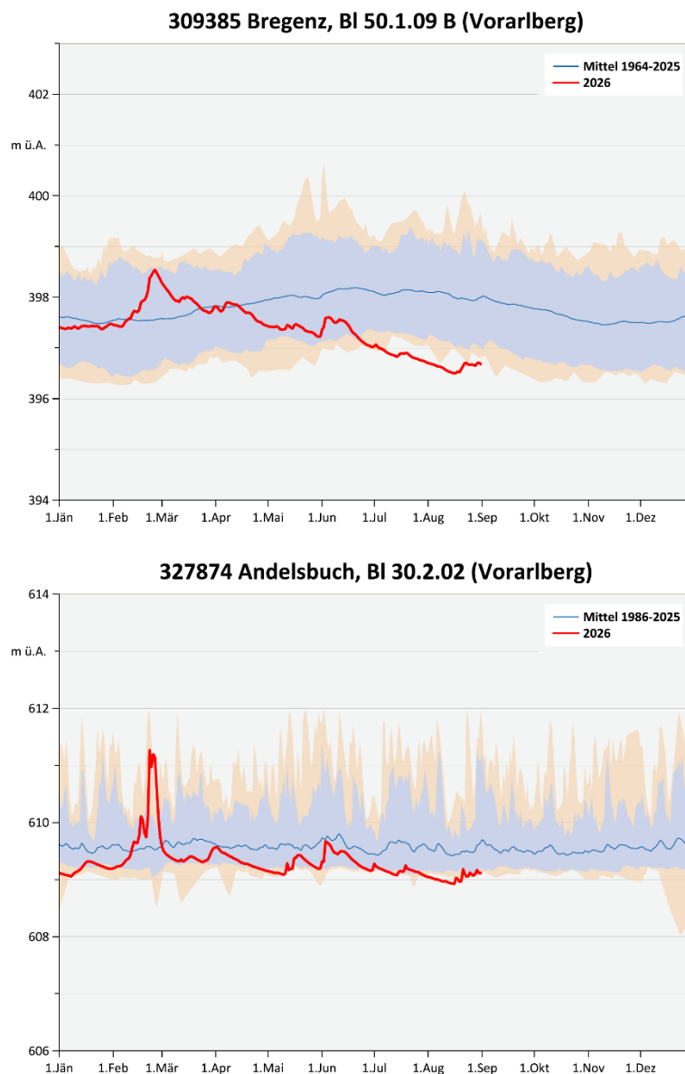
Abbildung 21. Tagesmittel des Grundwasserstandes 2026 (Rheintal, Bregenzer Wald, Montafon) im Vergleich zum langjährigen Tagesmittel; innerhalb der blauen Fläche liegen 90 Prozent der Tagesmittel, die orangenen Begrenzungen zeigen die Minima und Maxima.
