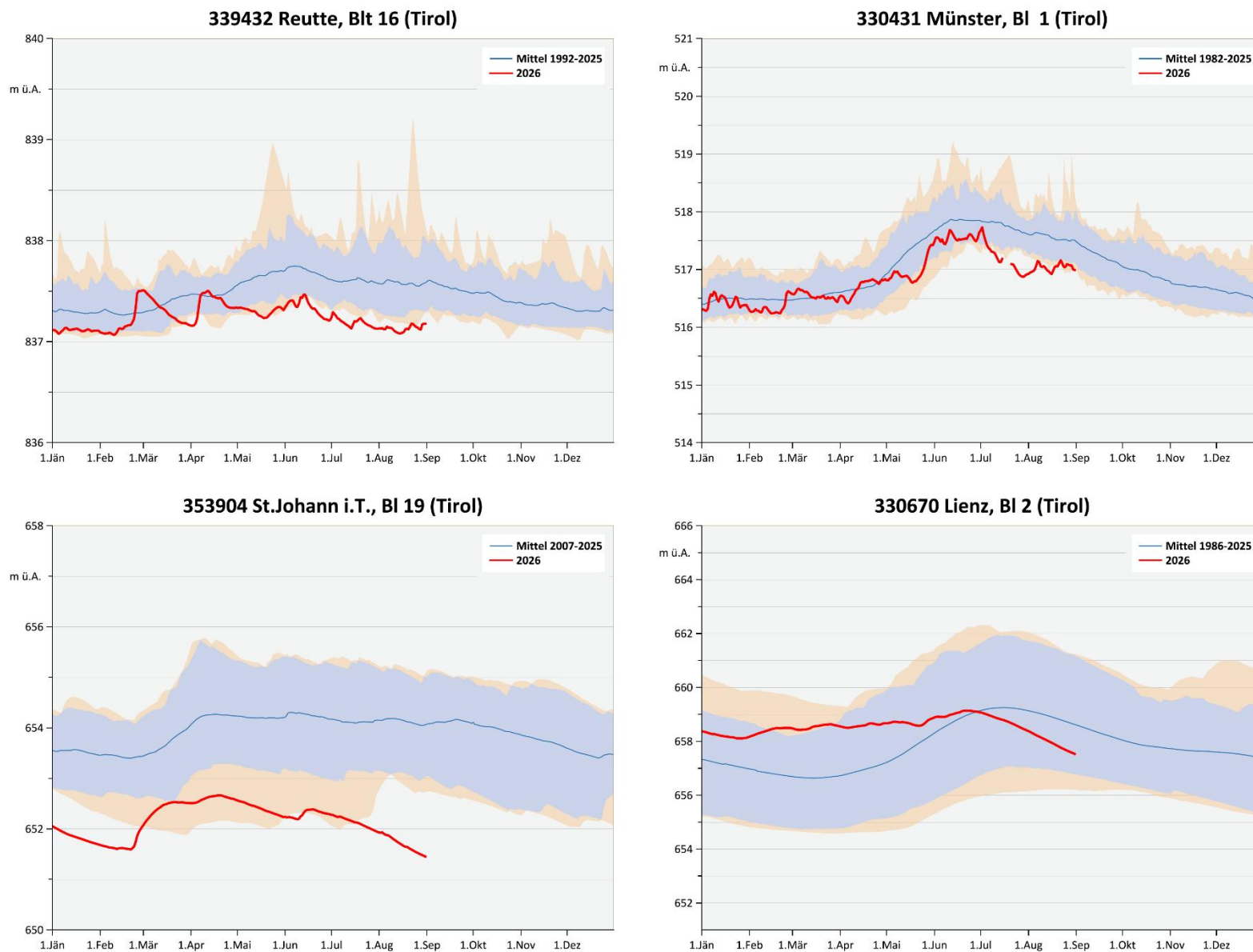
Abbildung 22. Tagesmittel des Grundwasserstandes 2026 (Unteres Lechtal, Unteres Inntal, Großachengebiet, Lienzener Becken) im Vergleich zum langjährigen Tagesmittel; innerhalb der blauen Fläche liegen 90 Prozent der Tagesmittel, die orangenen Begrenzungen zeigen die Minima und Maxima.
