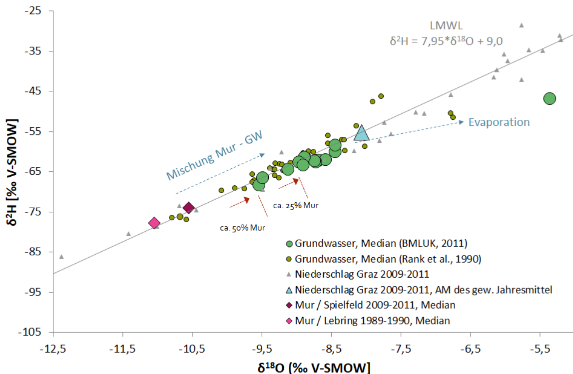
Abbildung 29: Mischungsdiagramm der stabilen Wasserisotope ( \delta^{18}\text{O} gegen \delta^2\text{H} ) zur Visualisierung der Isotopensignaturen von Grundwasser, Mur und Niederschlag im Grundwasserkörper Leibnitzer Feld [MUR].
