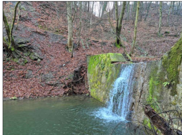
Abbildung 2: Konsolidierungssperre in hm 14,11
