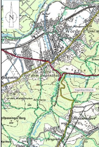
Abbildung 1: Einzugsgebiet Hagenbachklamm
