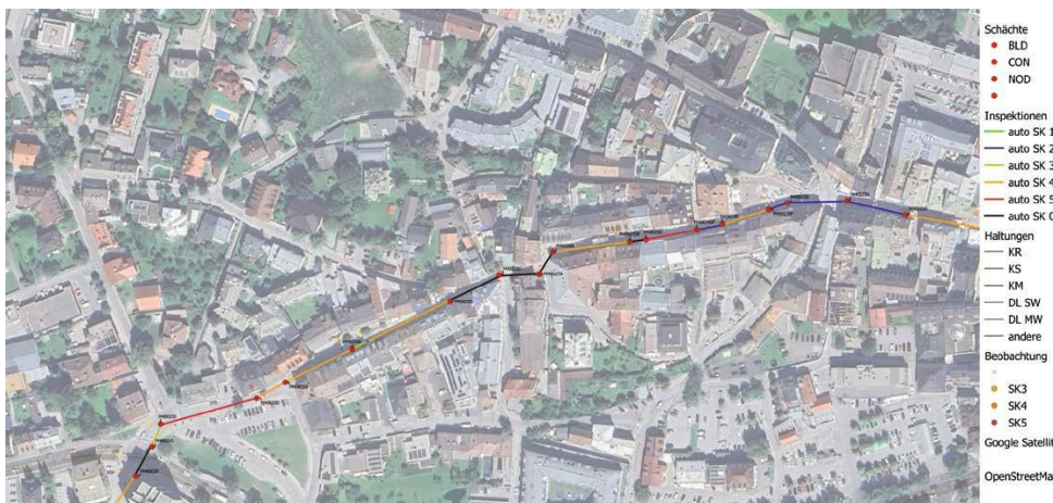
Lageplan eines Kanals mit Kennzeichnung der Schadensklassen
